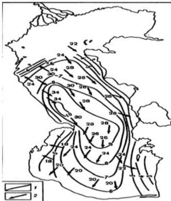
Рис. 4. Обобщённое экстремальное поле высот волн и скорости ветра [Атлас волнения и ветра Среднего и Южного Каспия, 1968].
